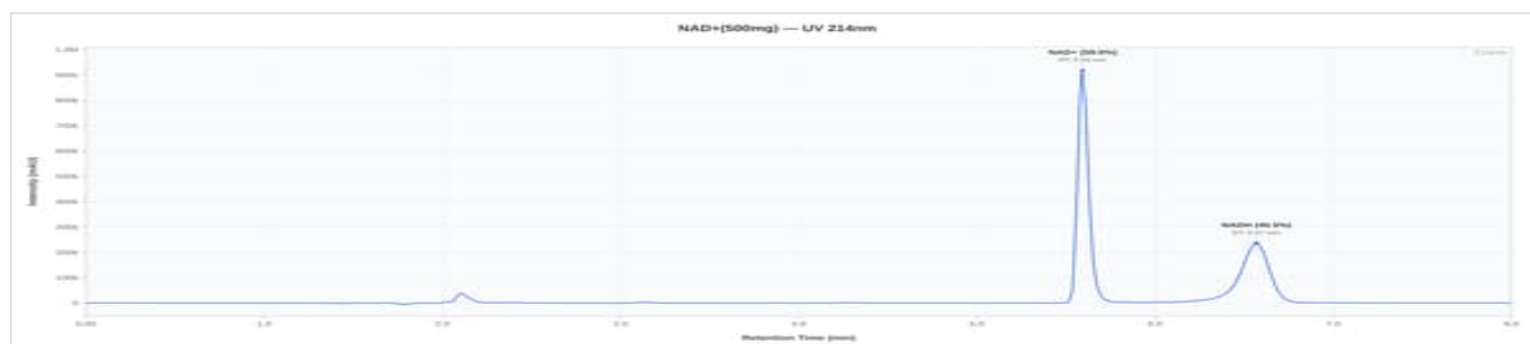
NAD+ 500mg - 001-B: UV Chromatogram
